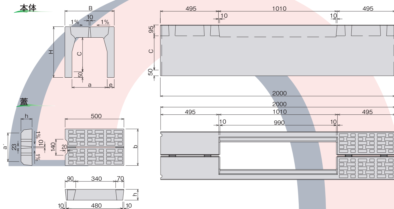
寸法表
