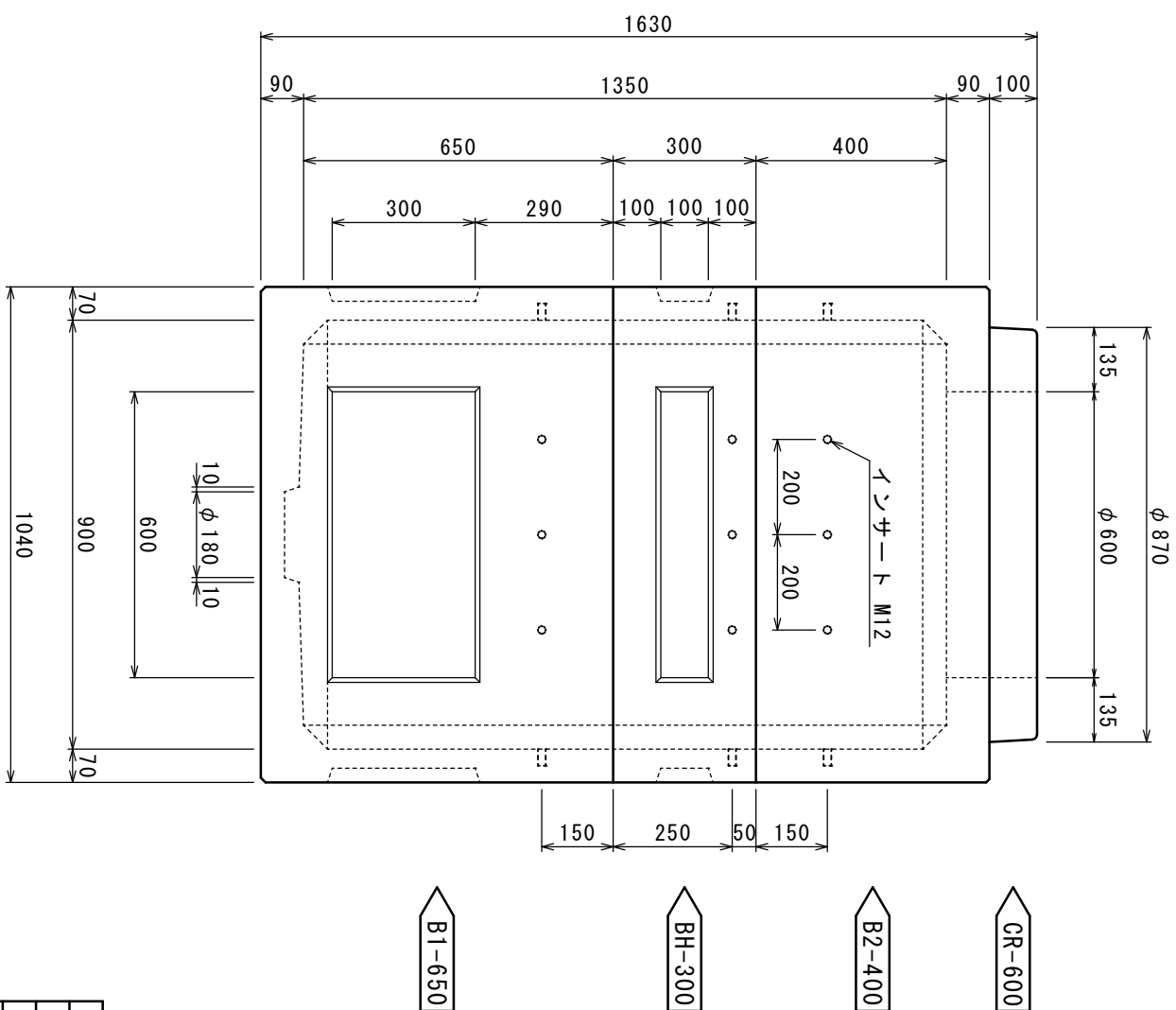
組立構造図
