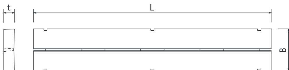
ディンプル側溝蓋 (表面：ファインステップ加工)
