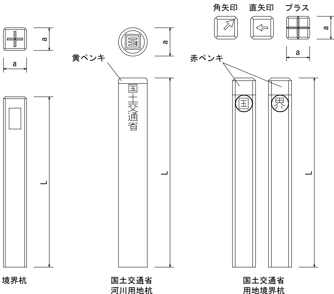
鉄筋コンクリート境界杭
